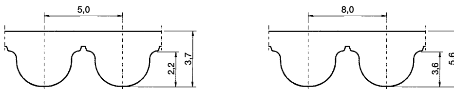
Конструкция полиуретановая со стальным кордом
