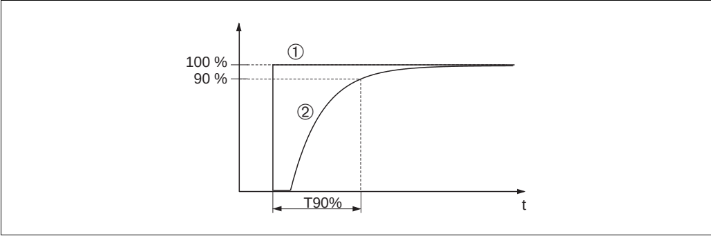
Представление времени реакции (T90%)
