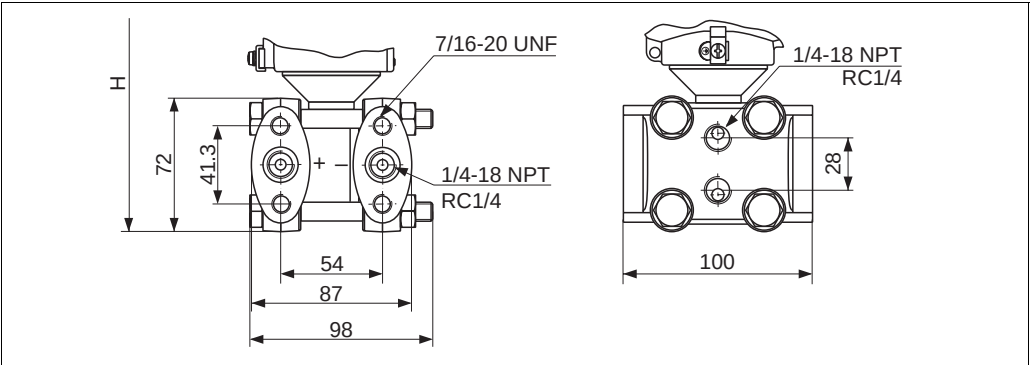
Подключение к процессу PMD 75, номинал ≥ 100 мбар
