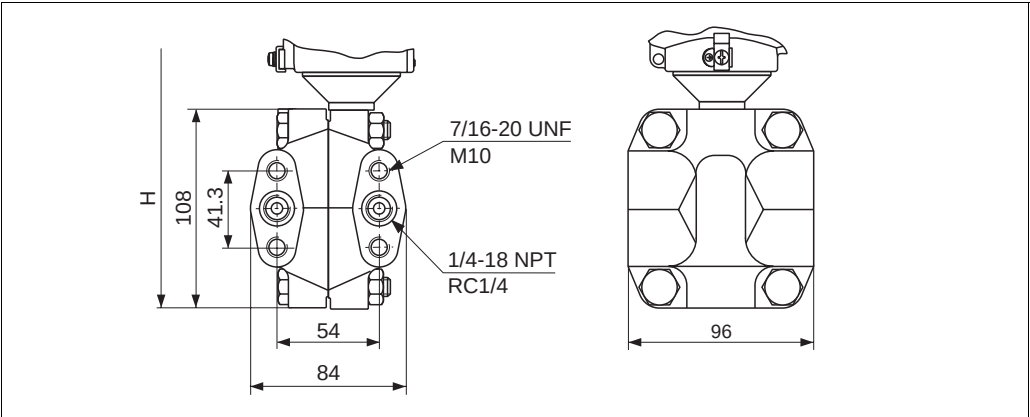
Подключение к процессу PMD 70, овальный фланец
