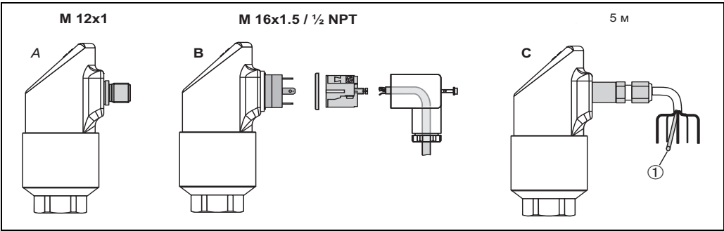
A: M 12x1 разъем; B: штепсель M 16x1.5 или 1/2 NPT C: кабель, 5 м длины, 5-контактный (→ подача справочного давления)
